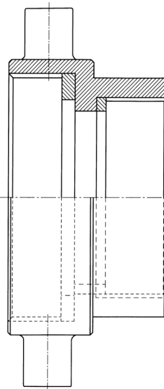
メスねじ
